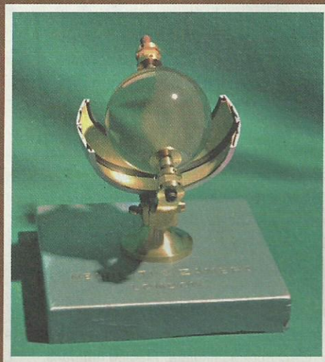
Figura 2 - Eliografano di Campbell
