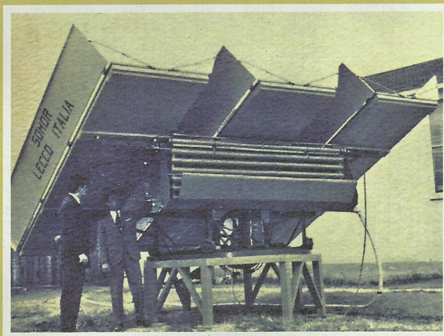
Pompa solare Somor presentata alla Conferenza di Tucson del 1954
